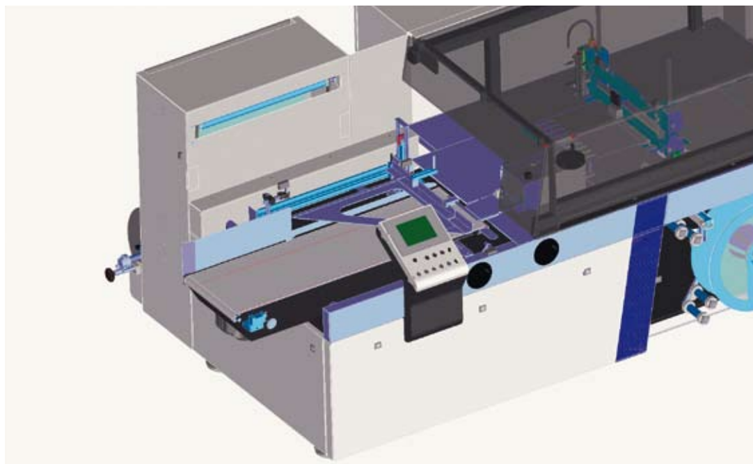
Version 1 : Alimentation par bande transporteuse intégrée dans la machine
