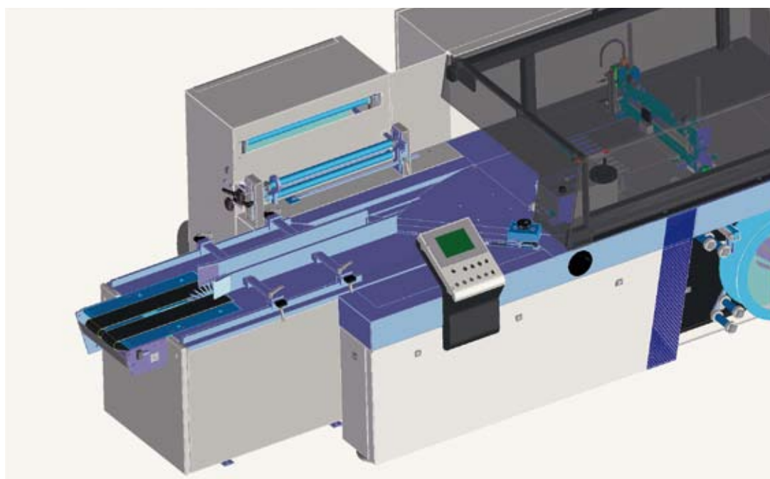
Version 2 : Alimentation par convoyeur à taquets intégré dans la machine
